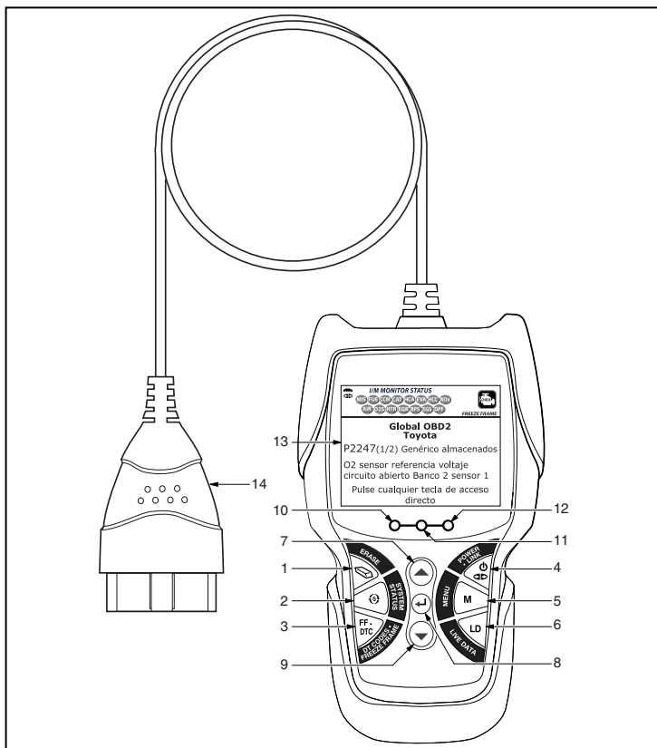
Figura 1. Controles y Indicadores
